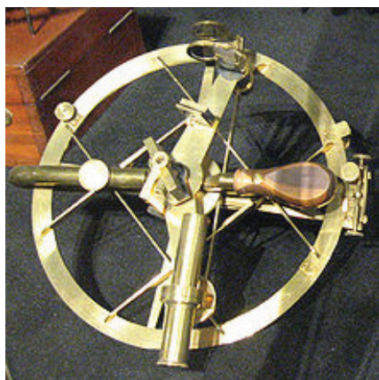
Instrument repetycyjny (koło powtarzające Borda lub inaczej koło Borda) – przyrządu takiego użyto do pomiarów południka. Przyrząd wynaleziony przez Etienne'a Lenoira w 1784 r., udoskonalony został przez Jeana Charles'a de Borda (1733–1799), matematyka, inżyniera i żeglarza.
