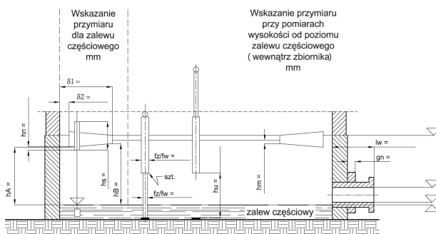
Rys. 3. Przykład schematu pierwszej cargi zbiornika z dachem pływającym
